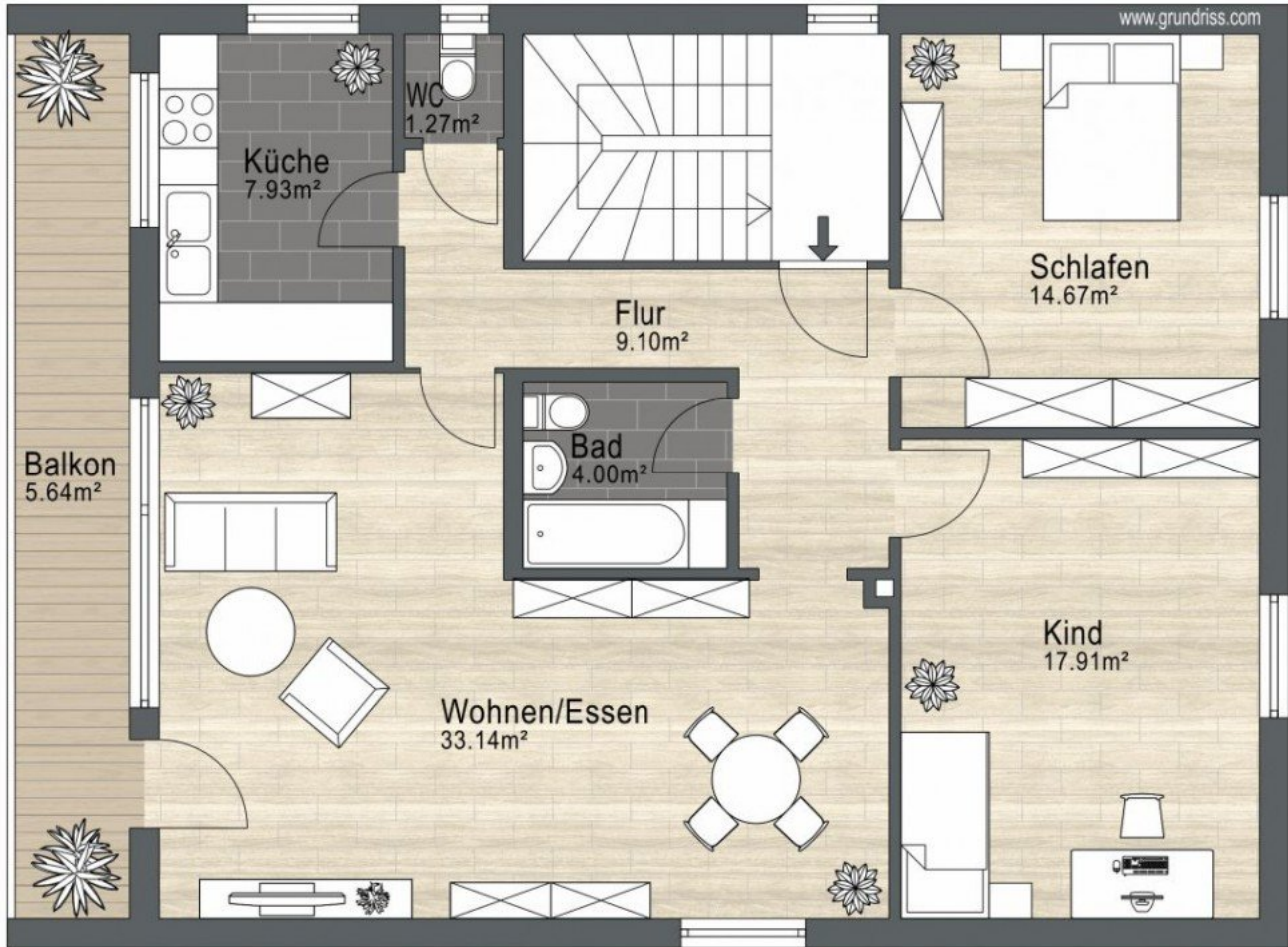
Grundriss
